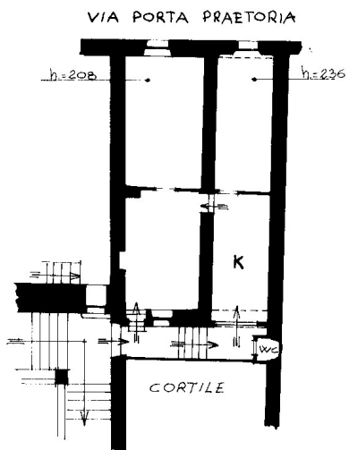
PIANTA PIANO PRIMO ALLOGGIO
