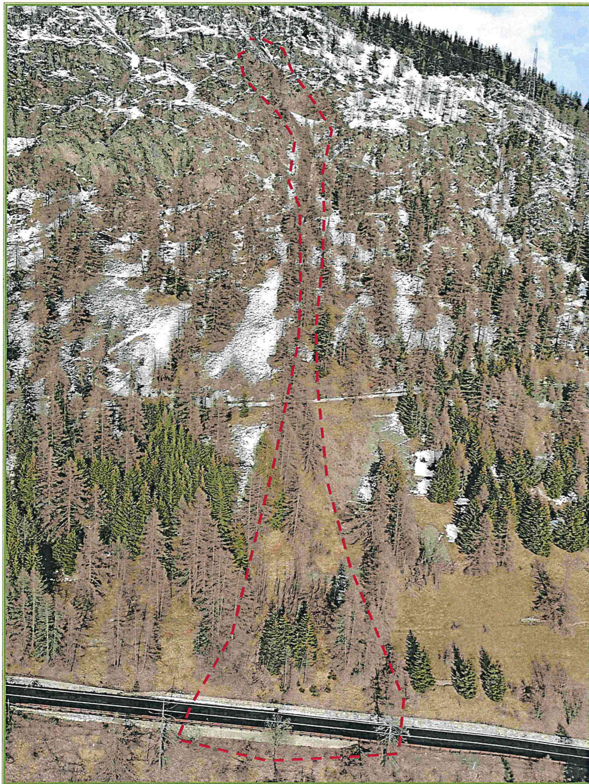
FOTO 1: vista frontale dall'elicottero della nicchia di distacco, del corridoio di caduta e il tratto di strada interessato dal crollo (S.S. n. 27 km da 21+000 a 21+200 circa)
