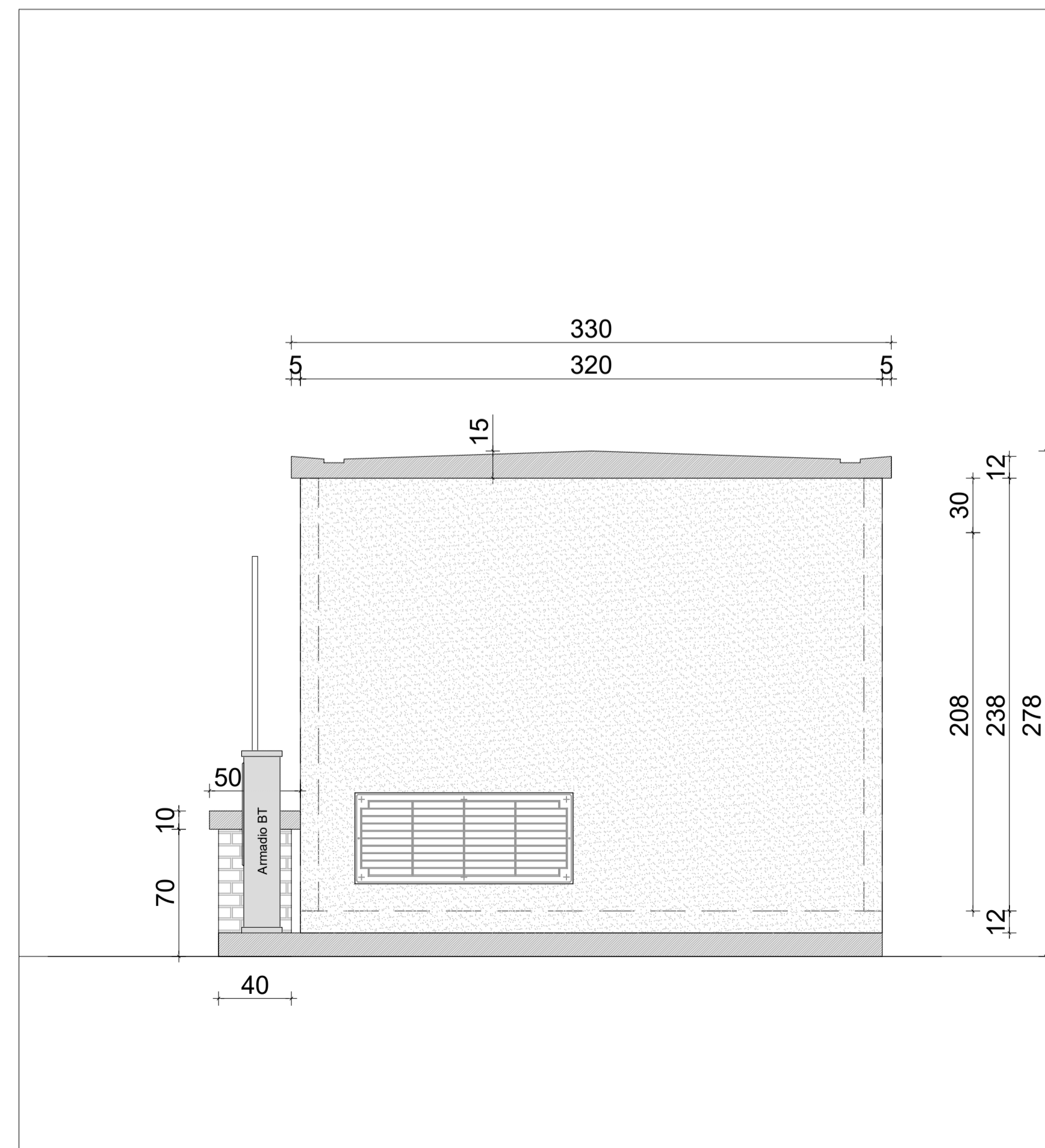
PROSPETTO EST - scala 1:25
