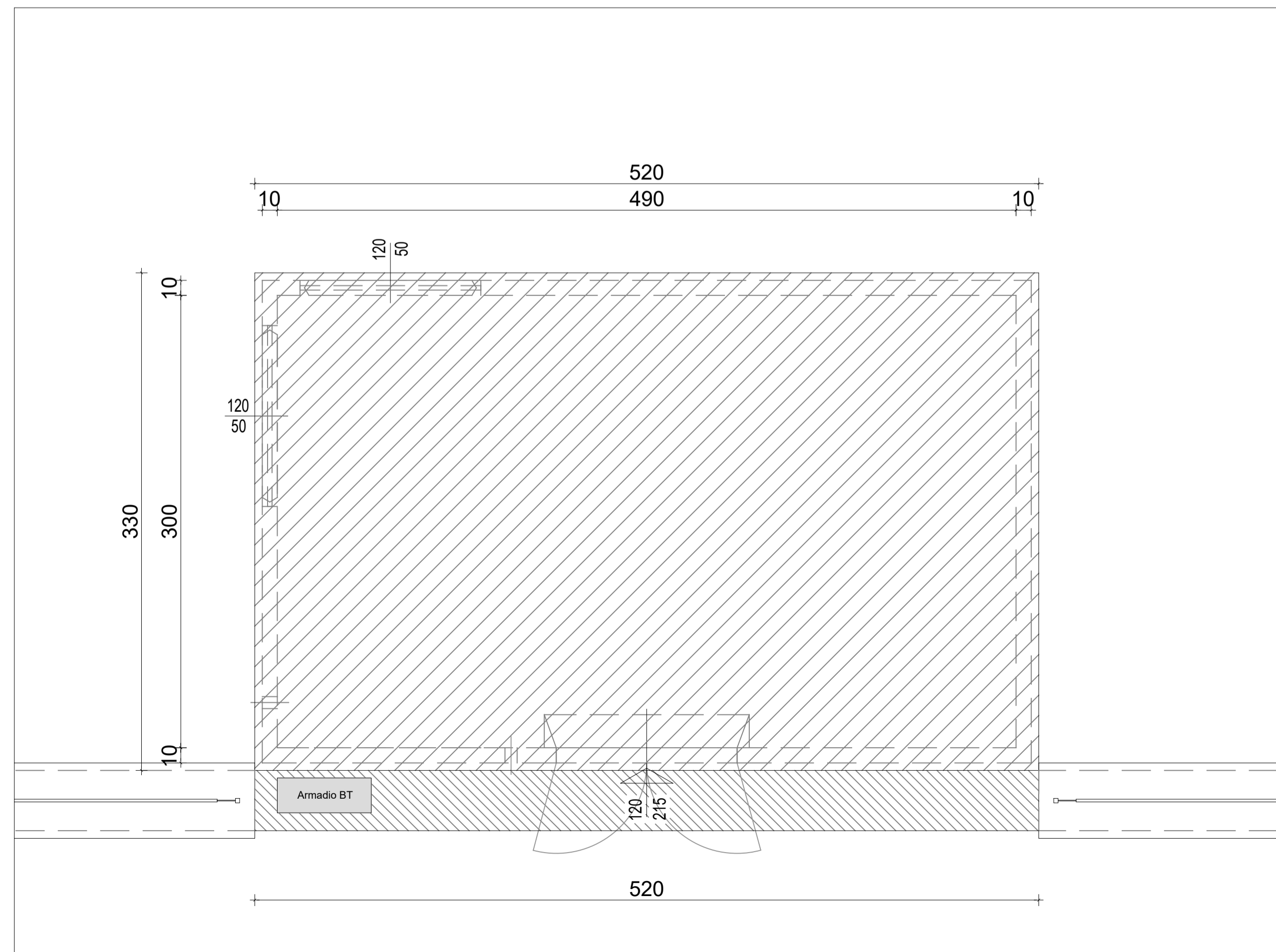
PIANTA - scala 1:25
