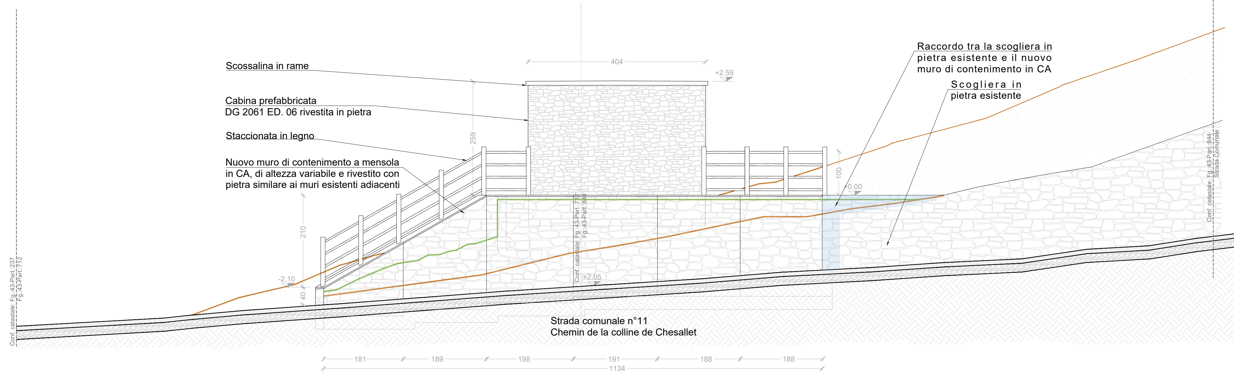
Prospetto Scala 1:50
