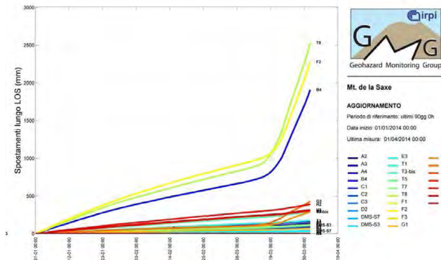
Figura 3.1 grafico complessivo dei prismi della rete di monitoraggio nel periodo 1/1/2014 – 31/3/2014.
