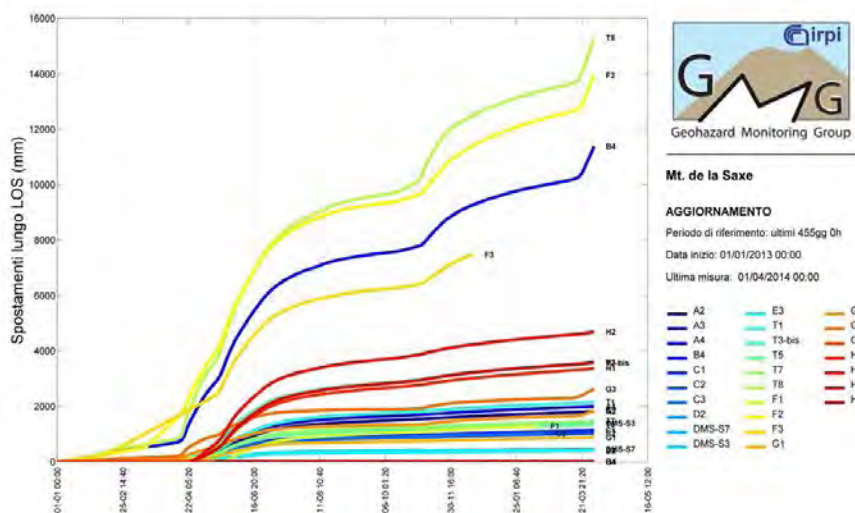
Figura 3.2 grafico dei prismi della rete di monitoraggio nel periodo 1/1/2013 - 31/3/2014
