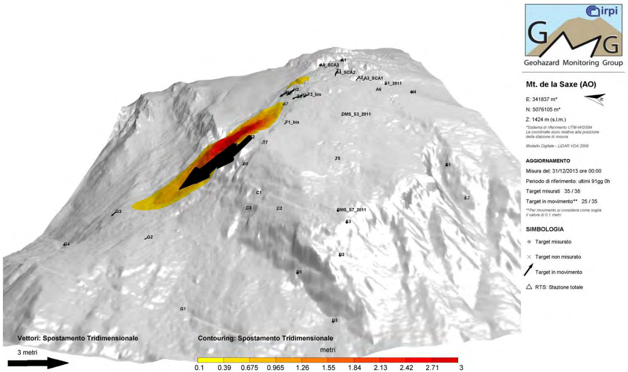
Figura 3.3 rappresentazione tridimensionale degli spostamenti cumulati nel trimestre di riferimento e nel trimestre precedente.
