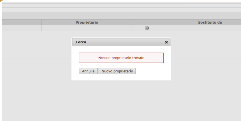
Figura 50 – Archivio ACE/APE
