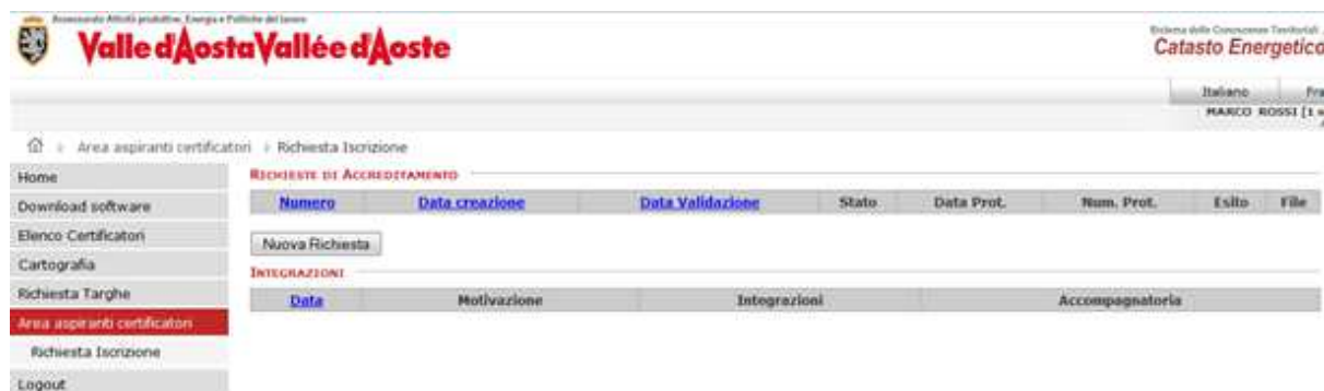
Figura 15 – richiesta iscrizione
