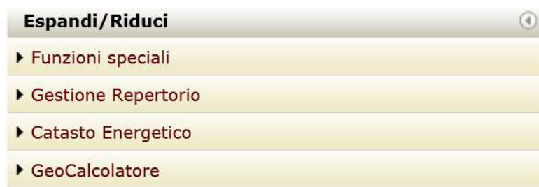
Figura 4 – menu funzioni
