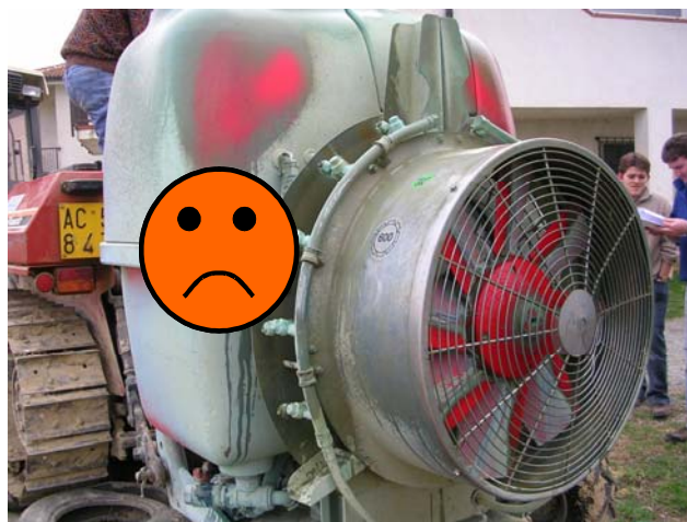
Fig. 23 – Macchina irroratrice sulla quale il getto prodotto dagli ugelli colpisce direttamente il serbatoio
