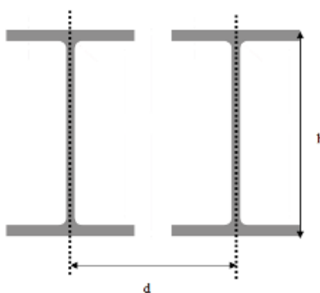
Figura C3.3.28 – Travi parallele
