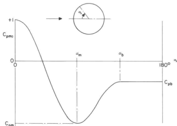
Figura C3.3.26 - Coefficiente di pressione esterna C_{pe}
