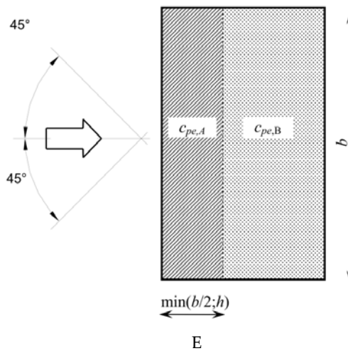
Figura C3.3.5 - Schema di riferimento per coperture piane
