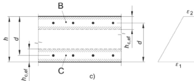
Figura C4.1.10- Area tesa efficace. Casi tipici
