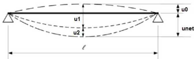
Figura C4.4.1 – Deformazione per un elemento inflesso
