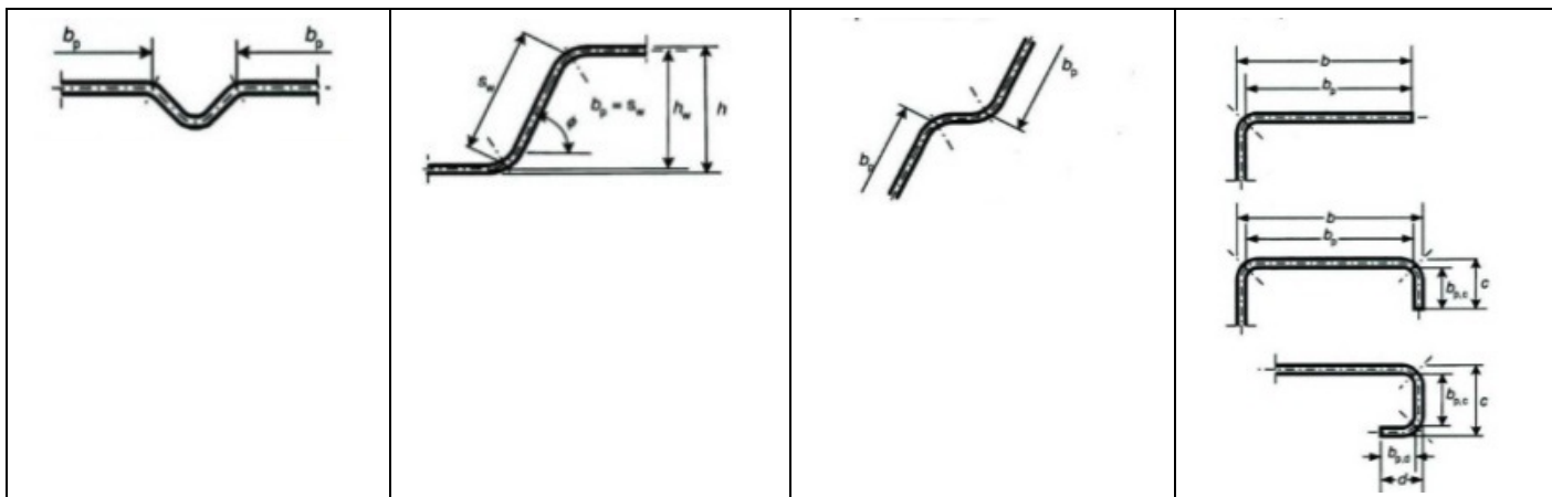
Figura C4.2.27 –Esempi di determinazione della larghezza b_p
