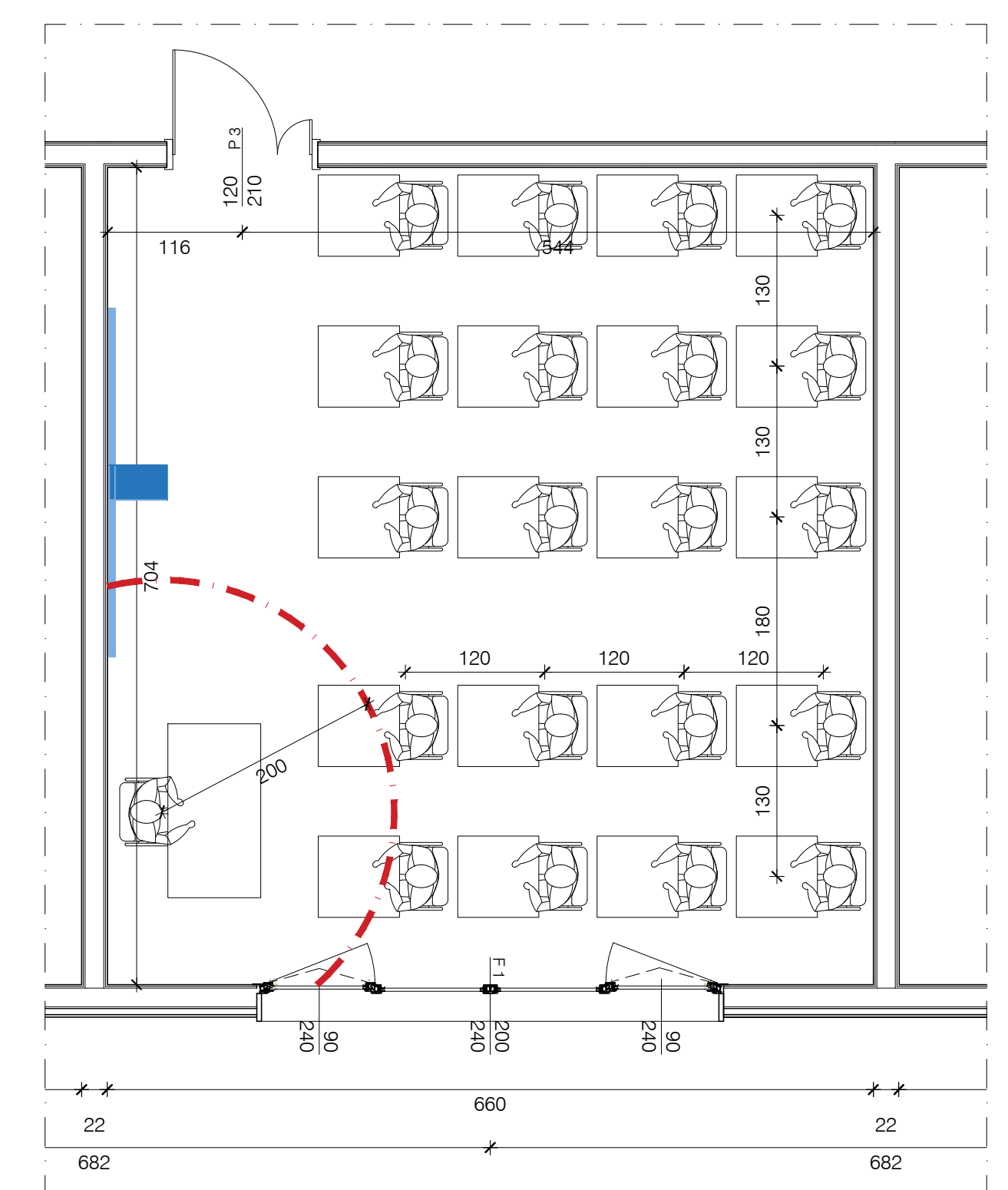
Pianta "aula tipo" scala 1:50
