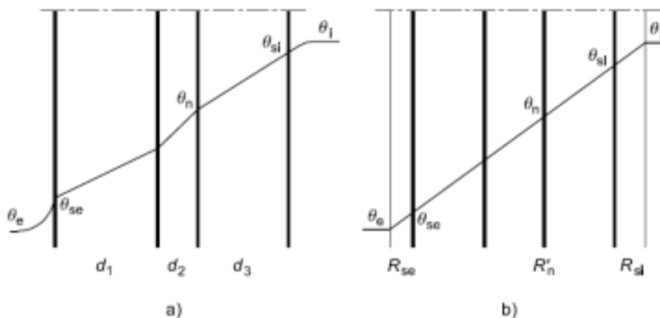
Figura 1 - Distribuzione di temperatura in un elemento edilizio multistrato (a) in funzione dello spessore di ogni strato e (b) in funzione della resistenza termica di ogni strato
