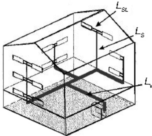
Figura C.6 - Definizione dei tratti di tubazione
