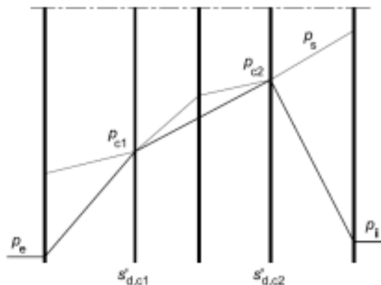
Figura 6 - Evaporazione da un componente edilizio nel caso in cui si sia verificata condensazione in due interfacce
