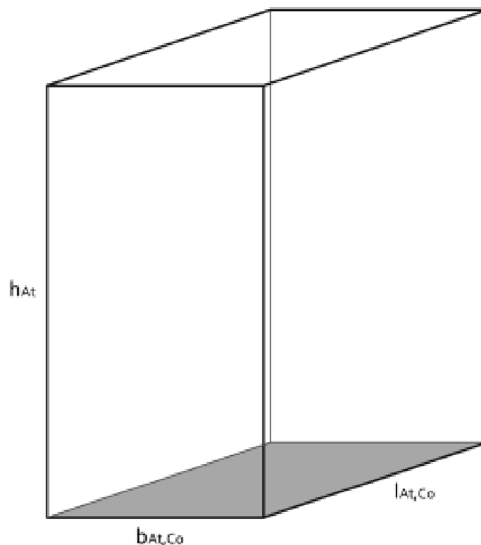
Figura 14 - Geometria di cortili ed atri
