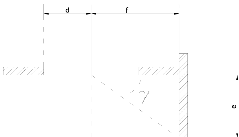
Figura 7 - Angolo di ombreggiamento di una superficie trasparente dovuto ad un aggetto verticale
