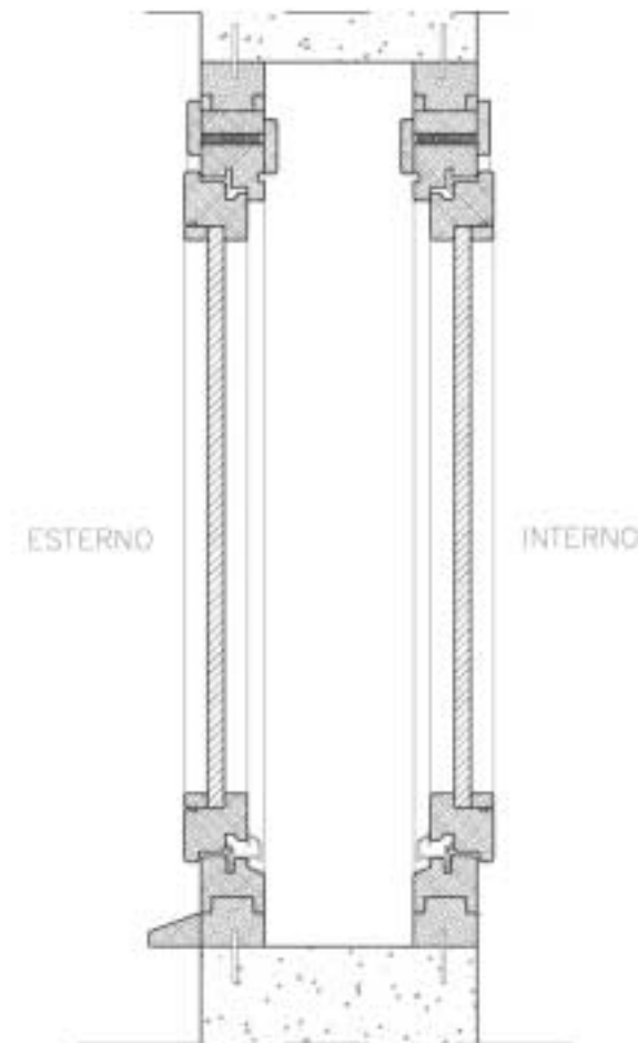
Figura 1 - Doppio serramento
