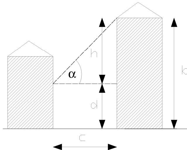
Figura 3 - Angolo di ombreggiamento di una superficie trasparente dovuto ad un'ostruzione esterna
