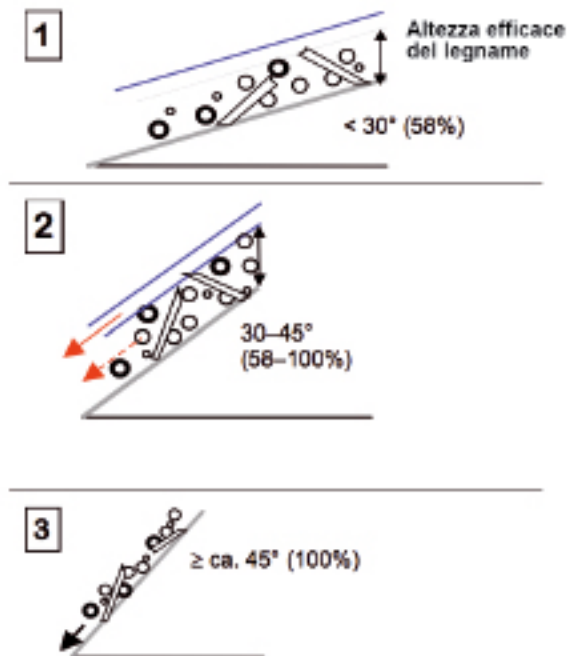
Figura 3.24 Stabilità della coltre nevosa in funzione della pendenza del terreno e dell'altezza efficace del legname abbandonato al suolo. (1) Con pendenze fino a 30° (58%) non bisogna temere il distacco di valanghe neppure se gli spessori della neve superano l'altezza efficace del legname di oltre 50 cm. (2) Con pendenze superiori a 30° (58%), e con una copertura di neve fresca che supera di 50 cm l'altezza utile del legname, sono da prevedere distacchi di valanghe. (3) In caso di pendenze ancora più ripide, lo strato di legname è talmente instabile al punto da mettersi in movimento anche senza un'ulteriore pressione della neve. A partire da pendenze superiori a circa 50° (120%) la neve si scarica progressivamente dai pendii, impedendo in tal modo la formazione di valanghe importanti (UFAM, 2008).
