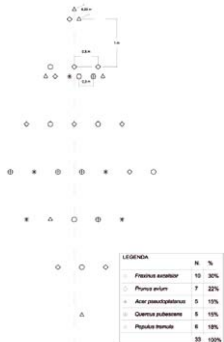
Figura 2.18 Schema di impianto per microcollettivi in una foresta di protezione diretta dalle valanghe a Valdieri (Cuneo) (progetto: M.Allocco, Seacoop S.r.l.).
