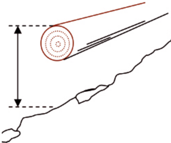
Figura 3.23 Con il termine di "altezza efficace" si indica l'elevazione media del punto superiore dei tronchi, misurata verticalmente rispetto al suolo. Si tratta della fascia all'interno della quale il legname disteso al suolo esercita un effetto stabilizzante sulla coltre nevosa, premesso comunque che l'altezza efficace non presenti lacune e sia ben distribuita all'interno delle zone più ripide di 30° (58%) (UFAM, 2008).
