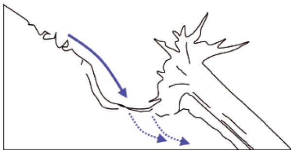
Figura 3.16 L'acqua superficiale può infiltrarsi nelle aperture del suolo provocate dallo sradicamento delle ceppaie e destabilizzarle (UFAM, 2008).
