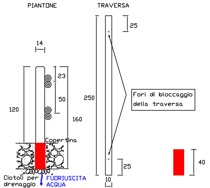
PIANTA DEI COMPONENTI
