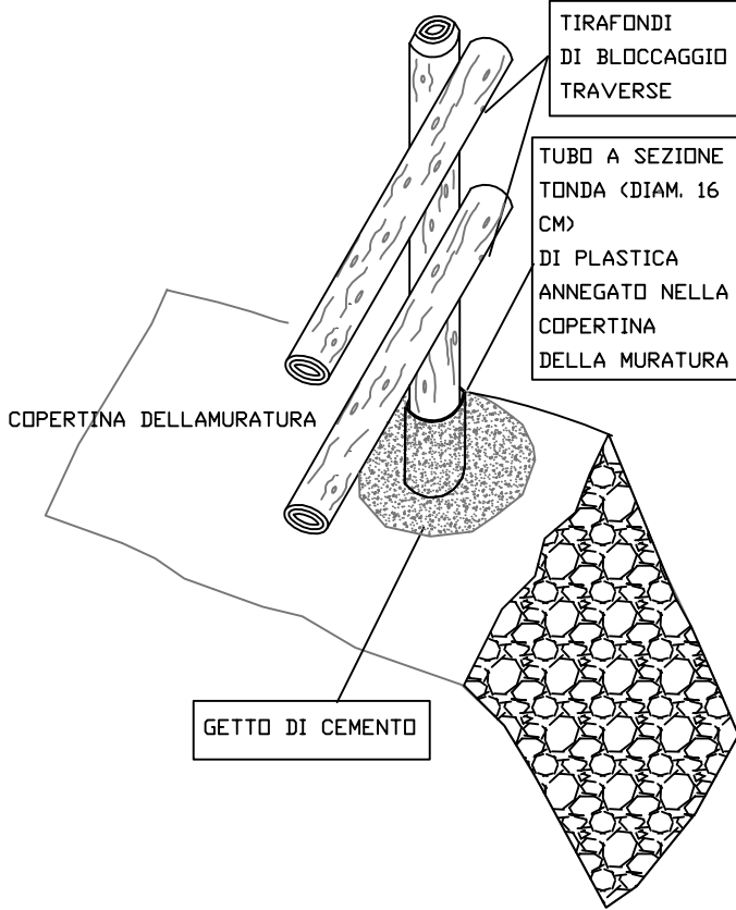
VISTA PROSPETTICA DI UN PIANTONE TERMINALE
