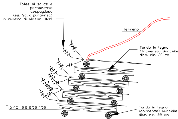
Sezione palificata doppia
