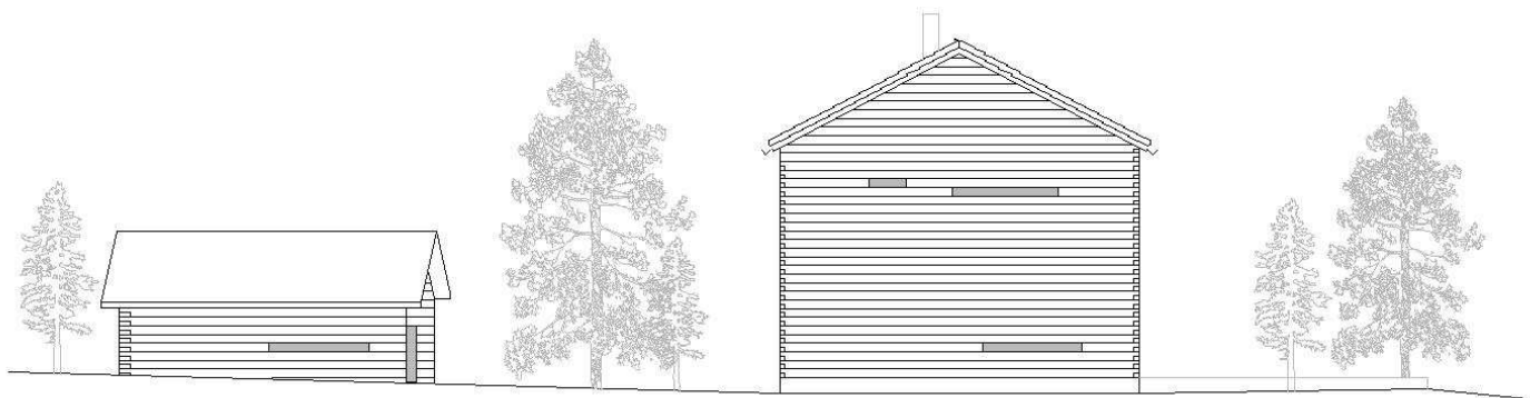
PROSPETTO NORD
